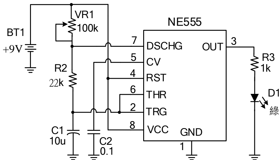
圖2、數位邏輯應用電路圖
