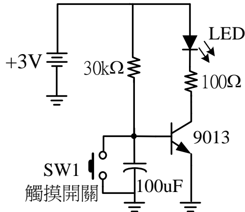
圖1、電晶體應用電路圖
