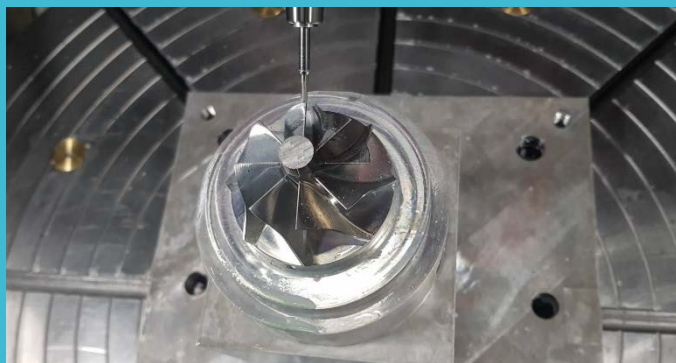
四軸車銑複 合加工機
