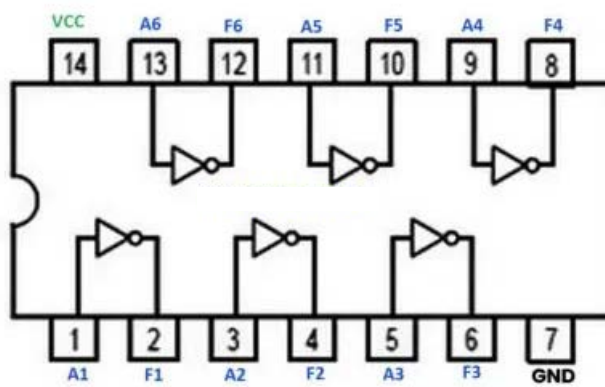
圖5、IC接腳圖
